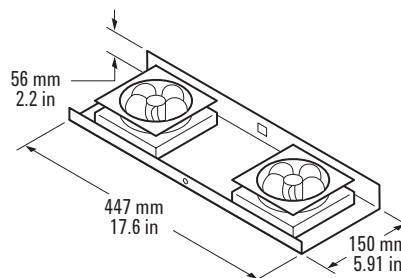
Extractor fan (E4470AZ)
